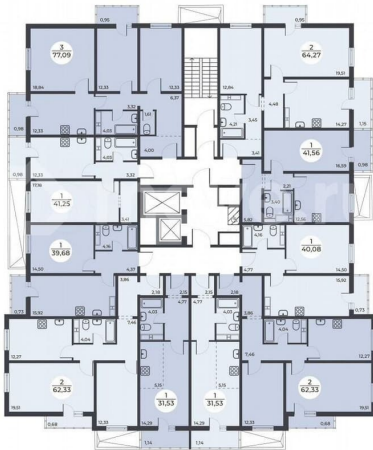
Типовой этаж
